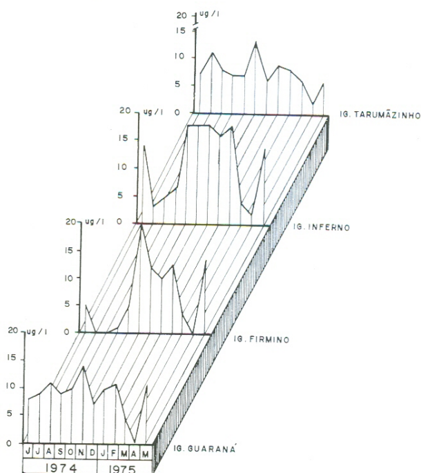
Fig. 8 — Variações mensais de nitrogênio de Kjeldahl.
