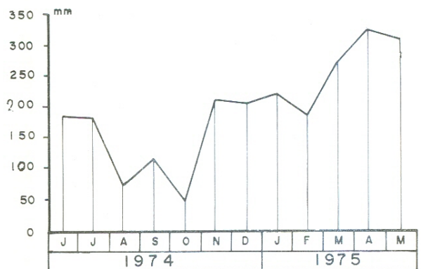
Fig. 5 — Dados de precipitação da Reserva Florestal Ducke. (Do Boletim Meteorológico do INPA 1974/1975, por gentileza da Chefe do Setor).
