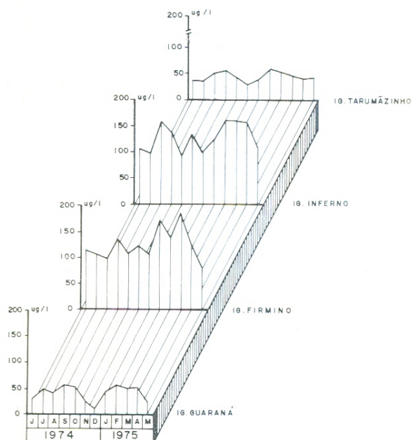
Fig. 2 — Variações mensais de nitrogênio amoniacal
