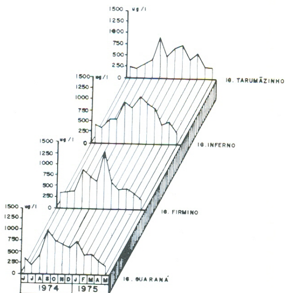
Fig. 7 — Variações mensais de nitrogênio total.
