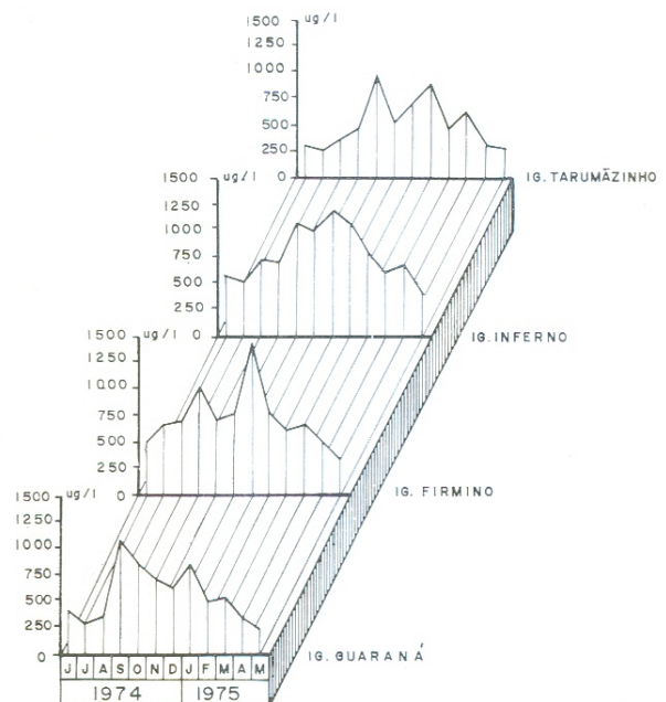
Fig. 6 — Variações mensais de nitrogênio orgânico.
