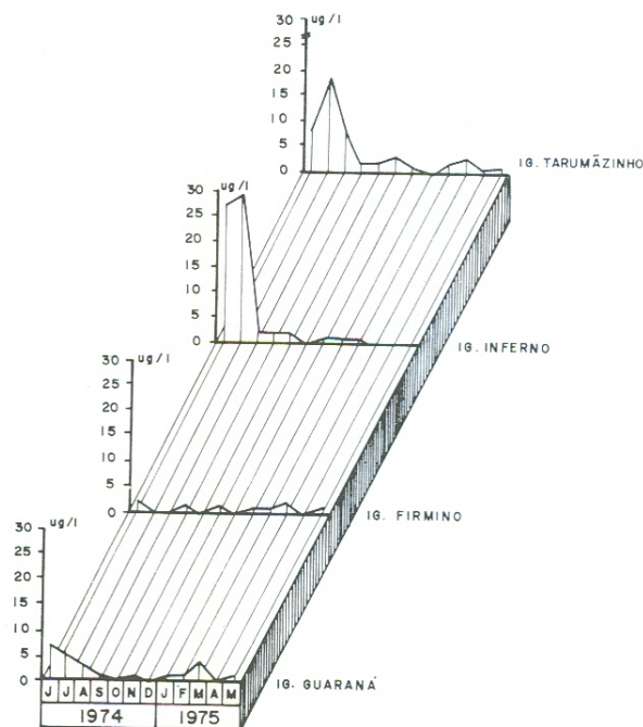
Fig. 4 — Variações mensais de nitrogênio na subfase dos nitratos.
