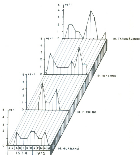
Fig. 3 — Variações mensais de nitrogênio na subfase dos nitritos.
