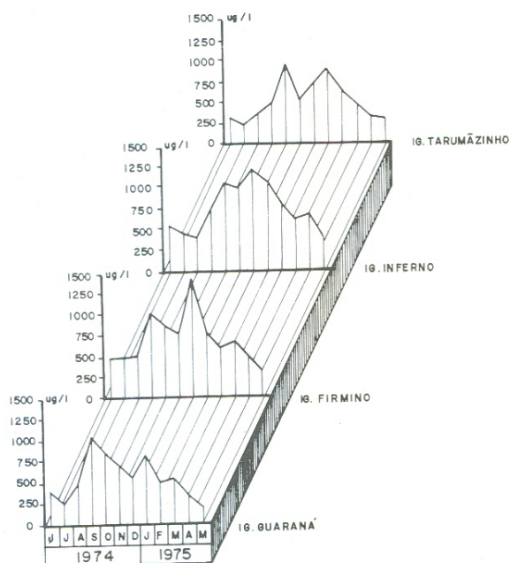
Fig. 9 — Variações mensais de fósforo.
